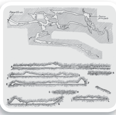
Fig. 3 Rilevamento topografico della cavità realizzato dalla Commissione Grotte della Società Alpina delle Giulie nel periodo ottobre-novembre 1926.
